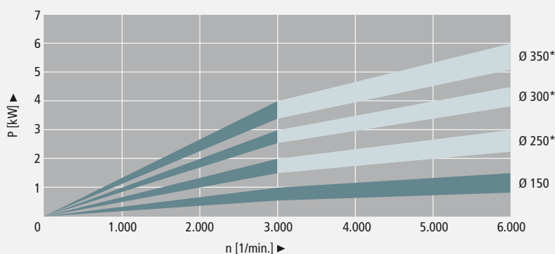
Leistungsbedarf einer Rundbürste
